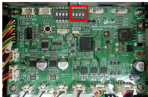
Рис. 55 Расположение DIP переключателя модуля ADVENT SOLID-700
