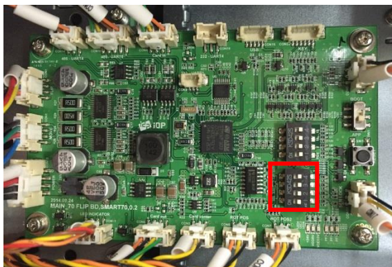
Рис. 55 Расположение DIP переключателя модуля ADVENT SOLID-700
