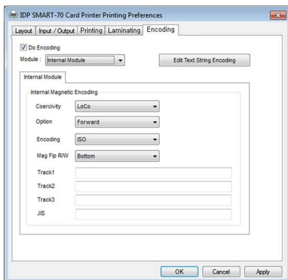
Рис. 85 Параметры кодировки
