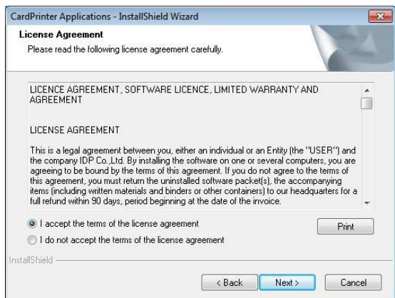
Рис. 76 Установка приложения
