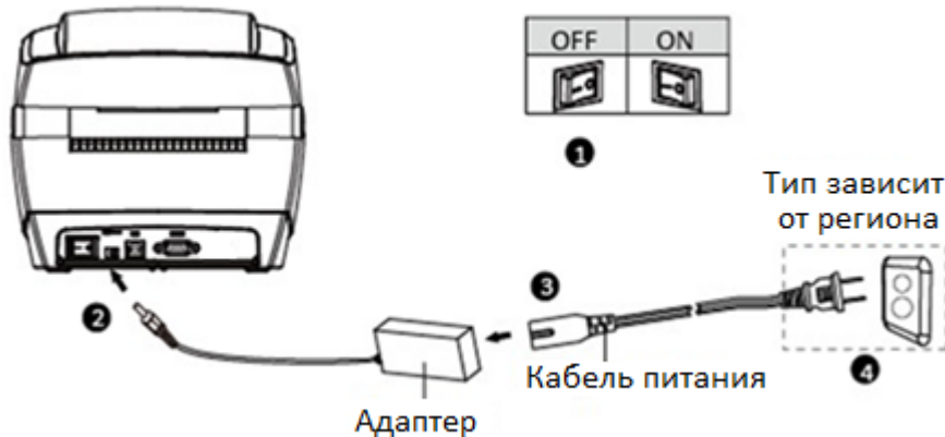
Рисунок 21. Подключение питания
