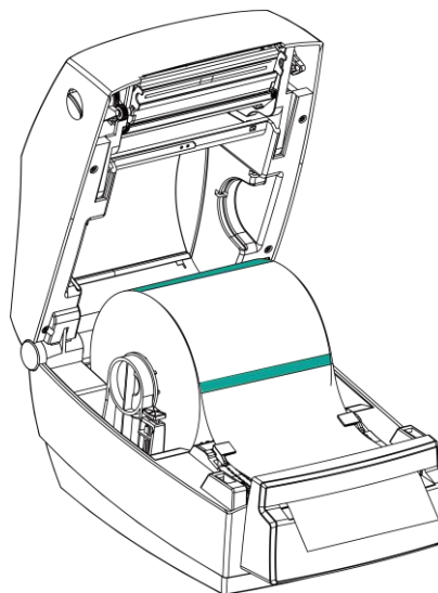
Рисунок 35. Протяжка этикет-ленты в щель модуля ножа
