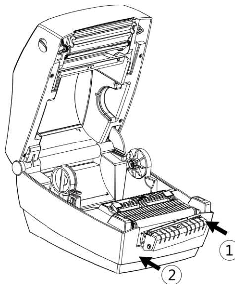
Рисунок 40. Установка отделителя
