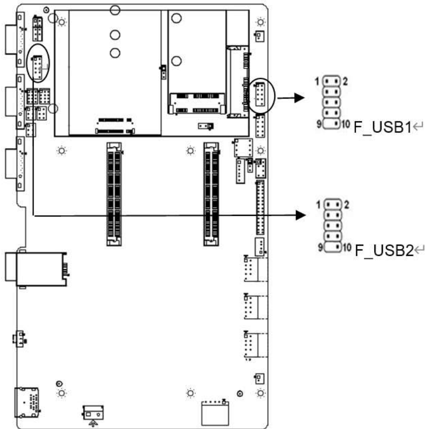
F_USB1、F_USB2
