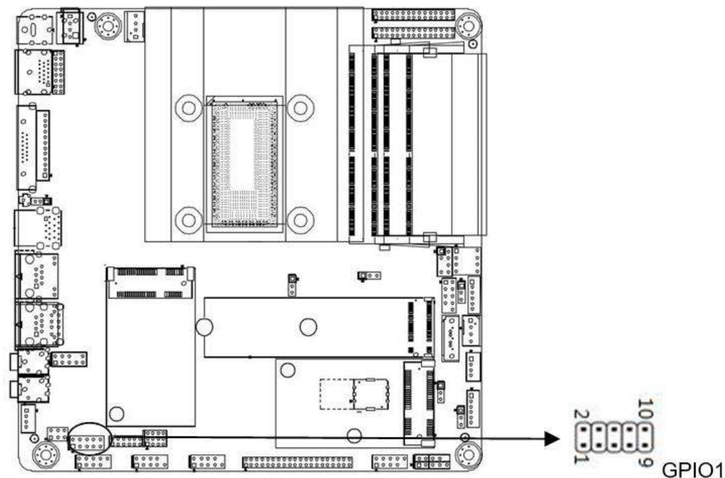
GPIO1 define
