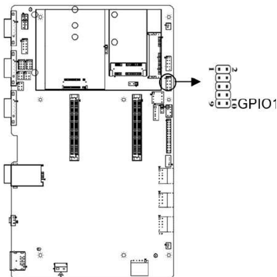
GPIO1 define
